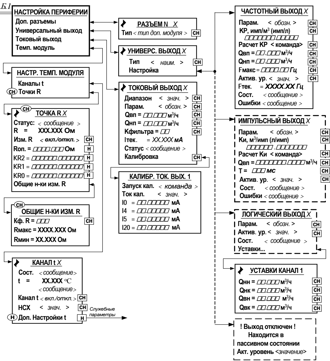
Рис.Б.5. Меню «Настройка периферии».
