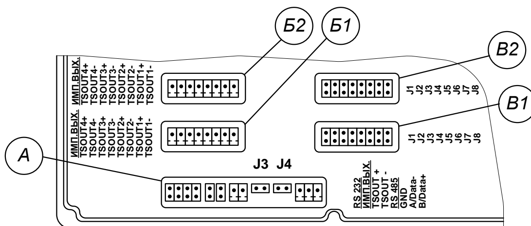
Рис.Ж.4. Коммутационные элементы модуля температурных входов
