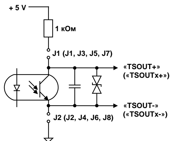
Рис.Е.1. Схема оконечного каскада универсальных выходов.
