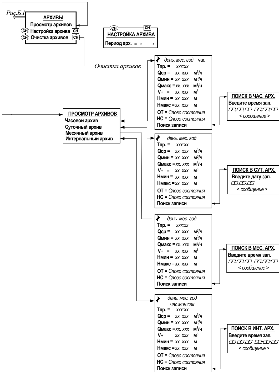
Рис.Б.7. Меню «Архивы».
