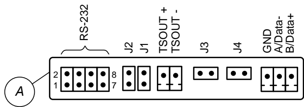
Рис.Ж.2. Коммутационные элементы комбинированного модуля.
