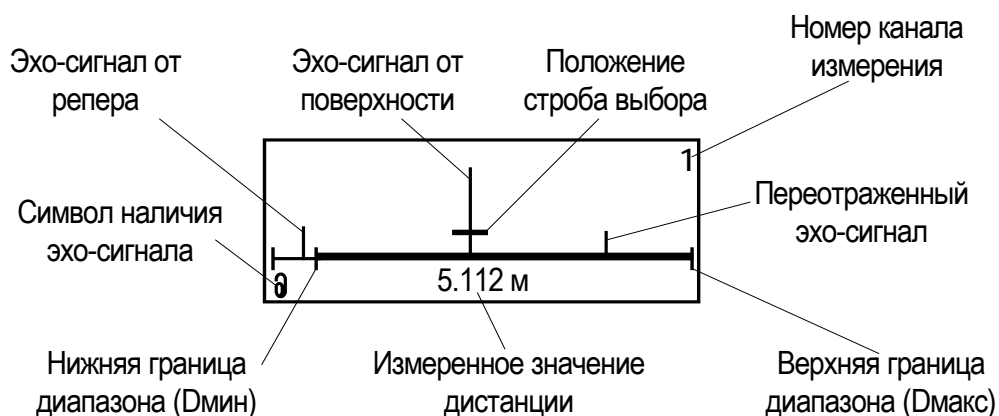
Рис. 4. Вид окна РАЗВЕРТКА.
